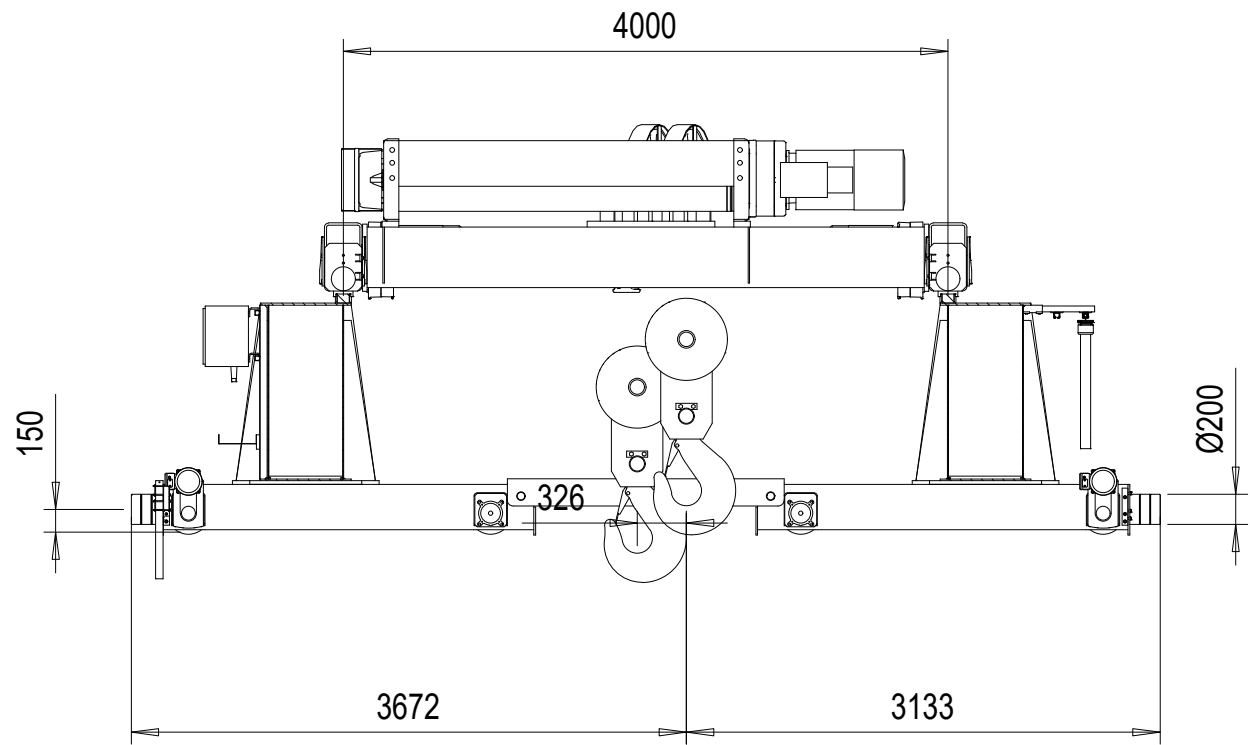
VIEW A-A
